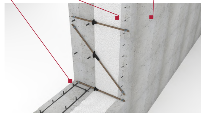
Композитный стержень со сплошным песчаным покрытием
